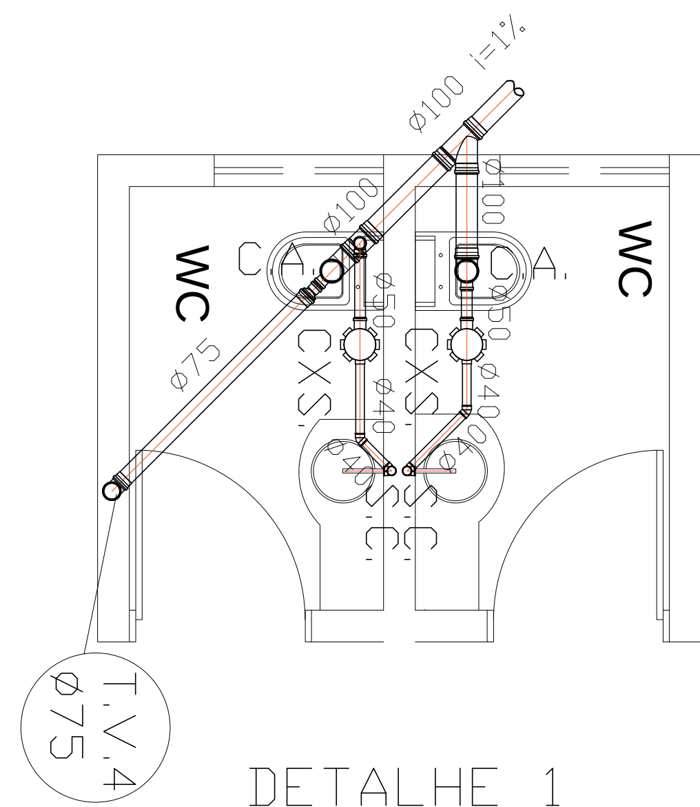
DETALHE 1 ESC. -----1/25
