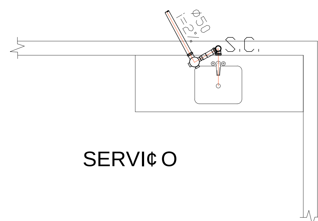
DETALHE 4 ESC. -----1/25
