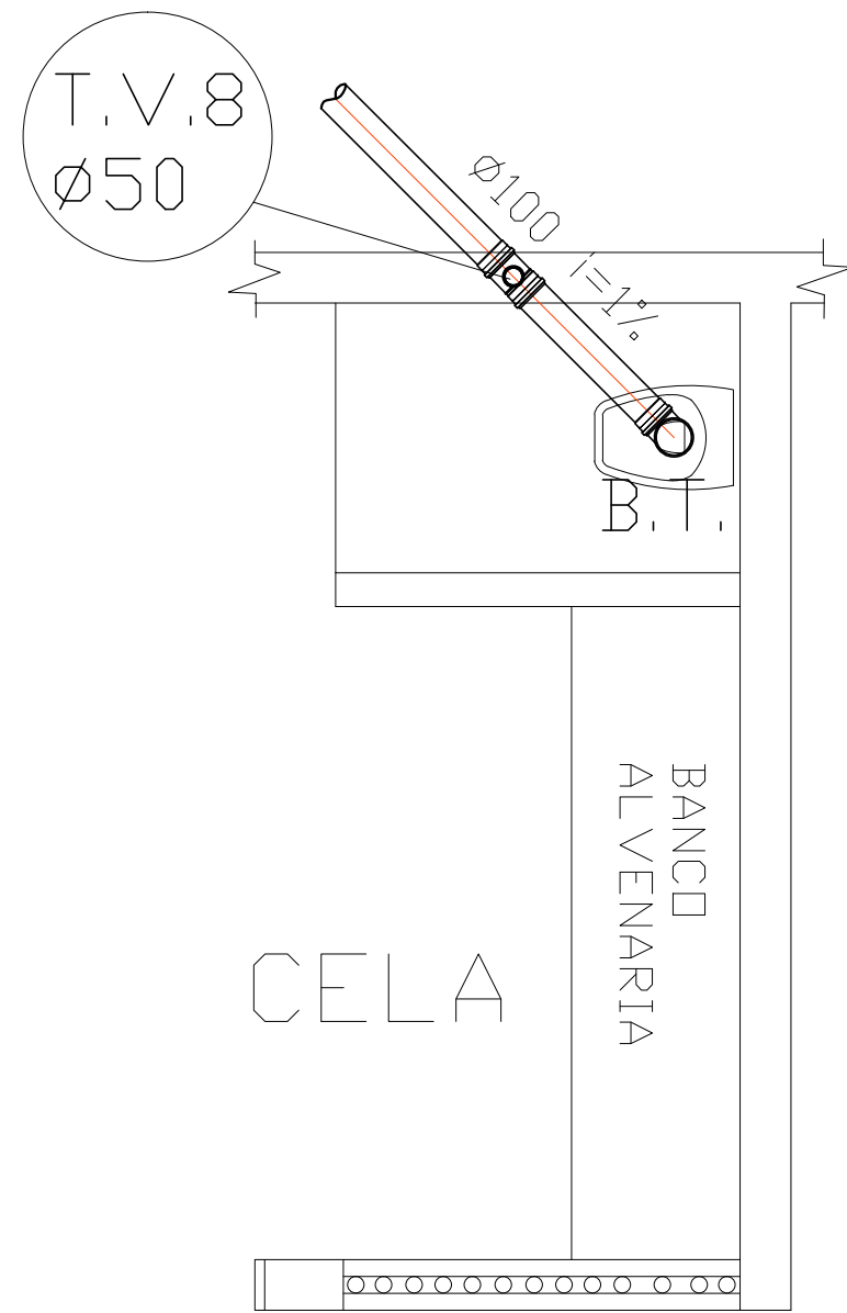
DETALHE 7 ESC. -----1/25
