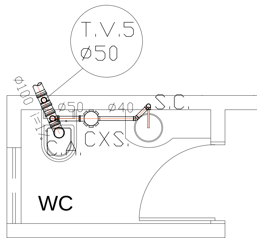
DETALHE 2 ESC. -----1/25
