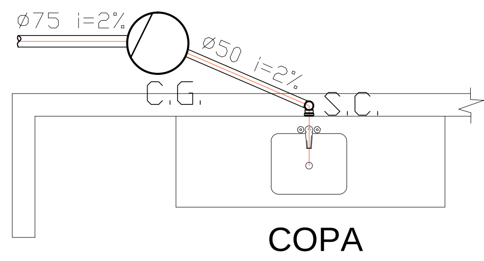
DETALHE 3=15 ESC. -----1/25
