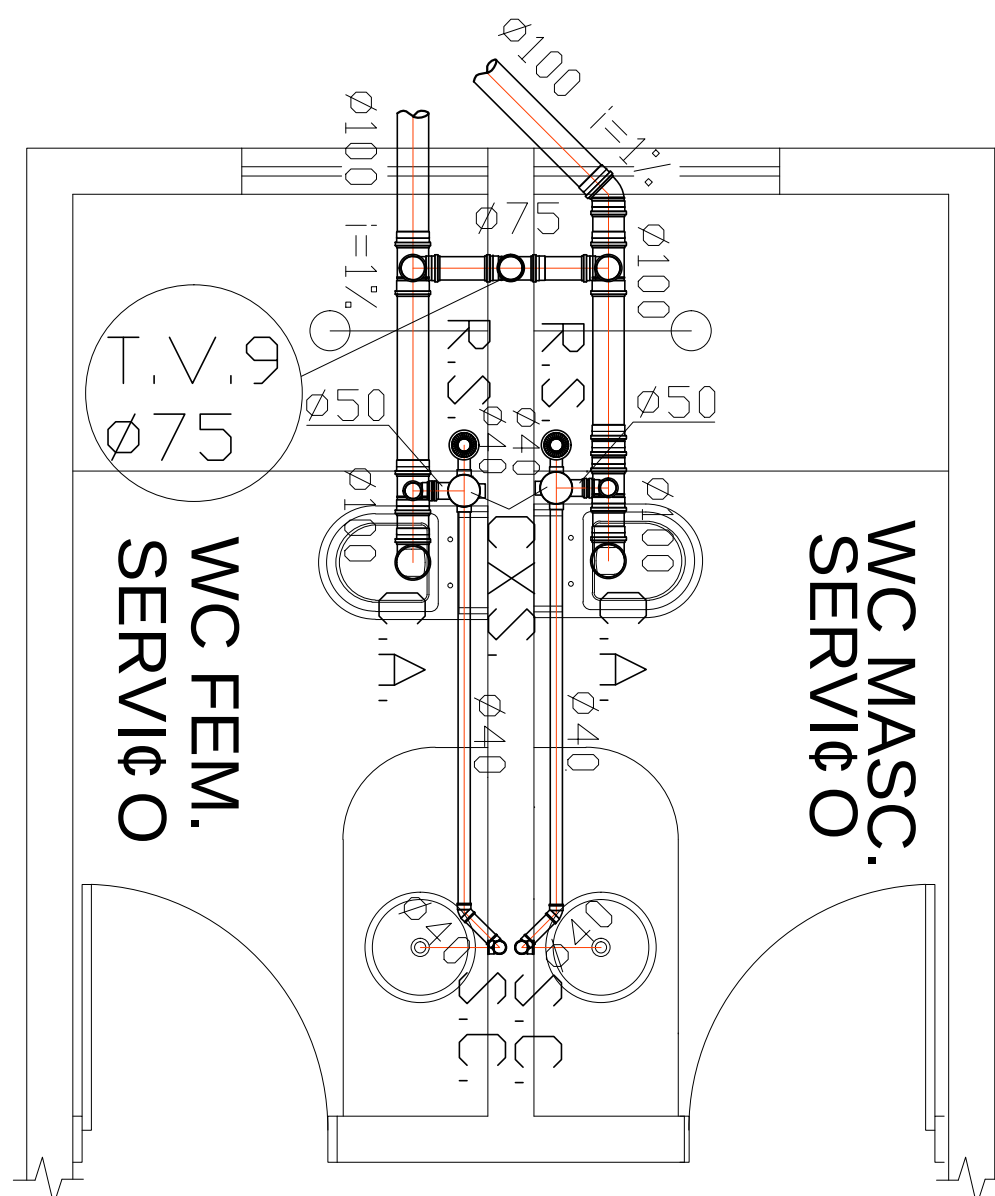
DETALHE 6 ESC. -----1/25
