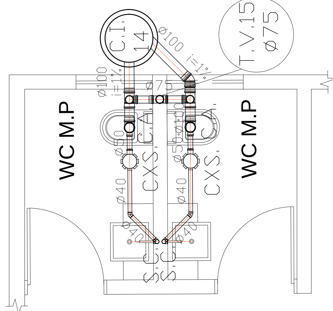
DETALHE 10 ESC. -----1/25
