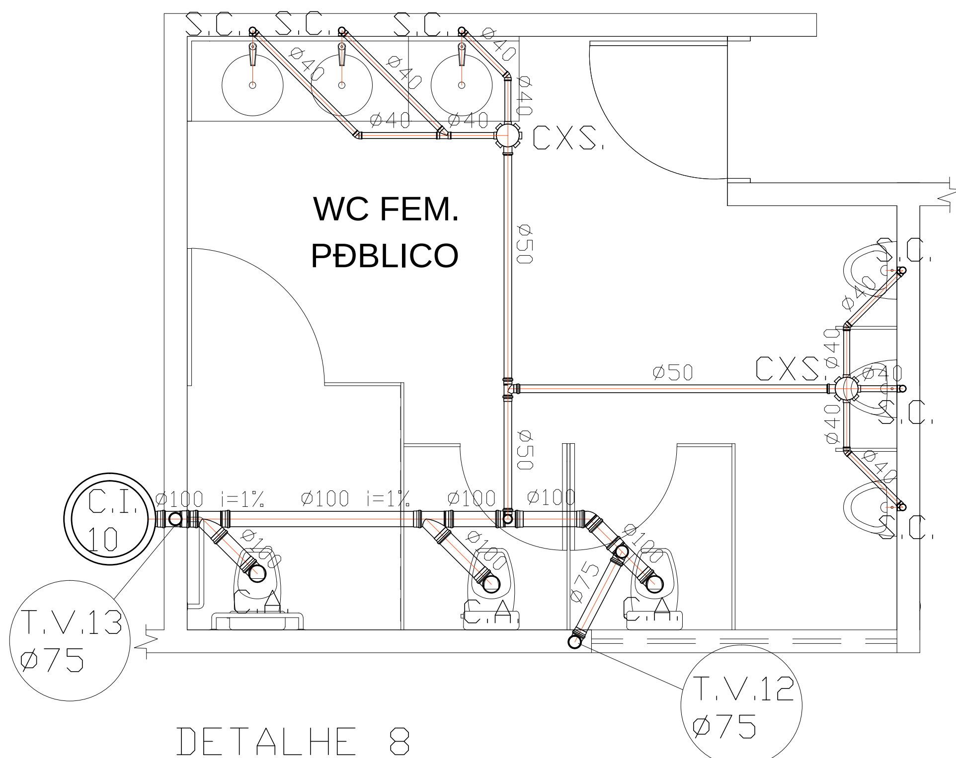
DETALHE 8 ESC. -----1/25
