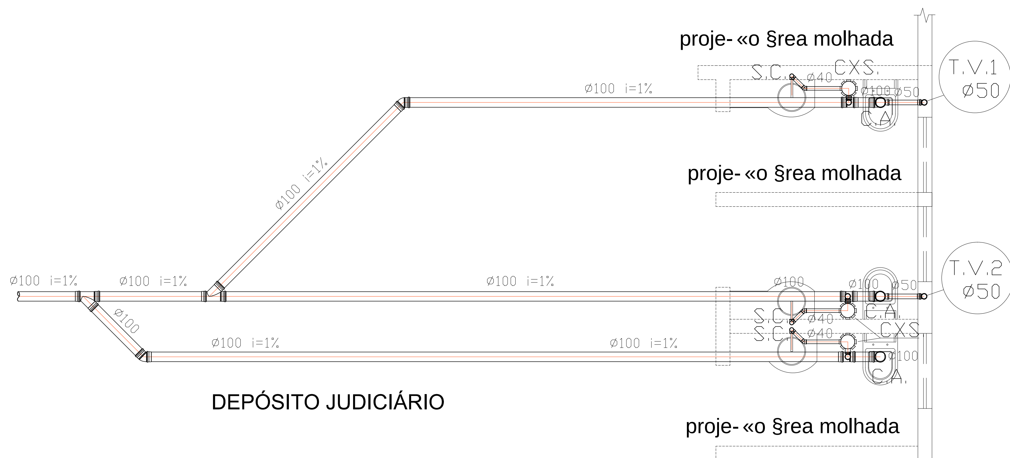
DETALHE 14 ESC. -----1/25
