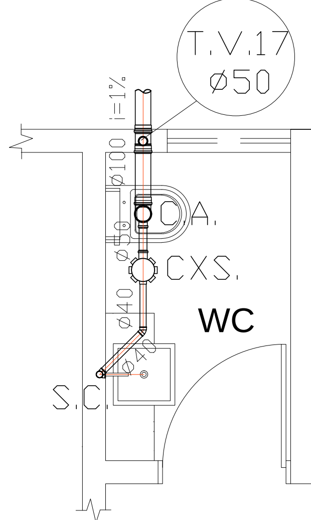
DETALHE 12 ESC. -----1/25
