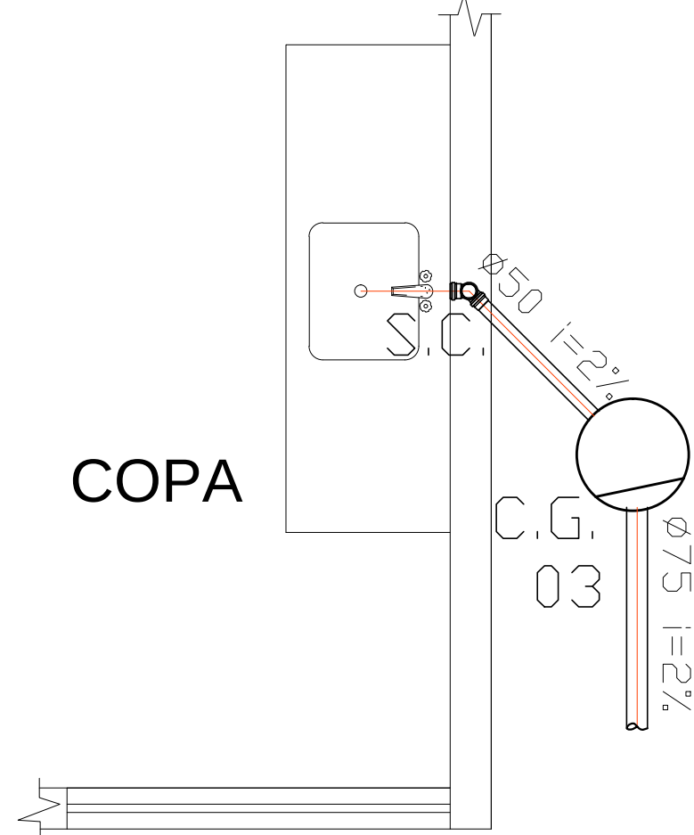
DETALHE 13 ESC. -----1/25
