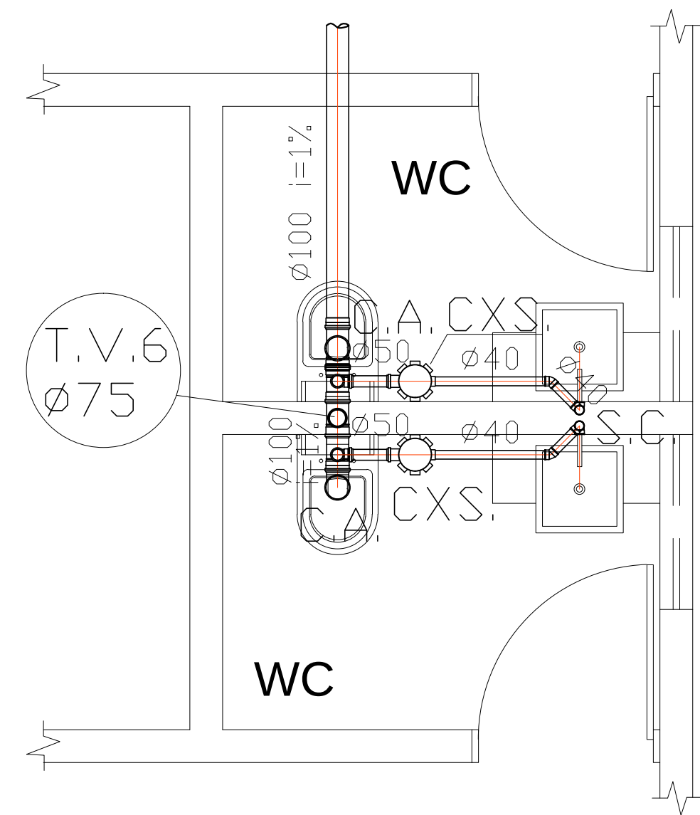
DETALHE 5 ESC. -----1/25
