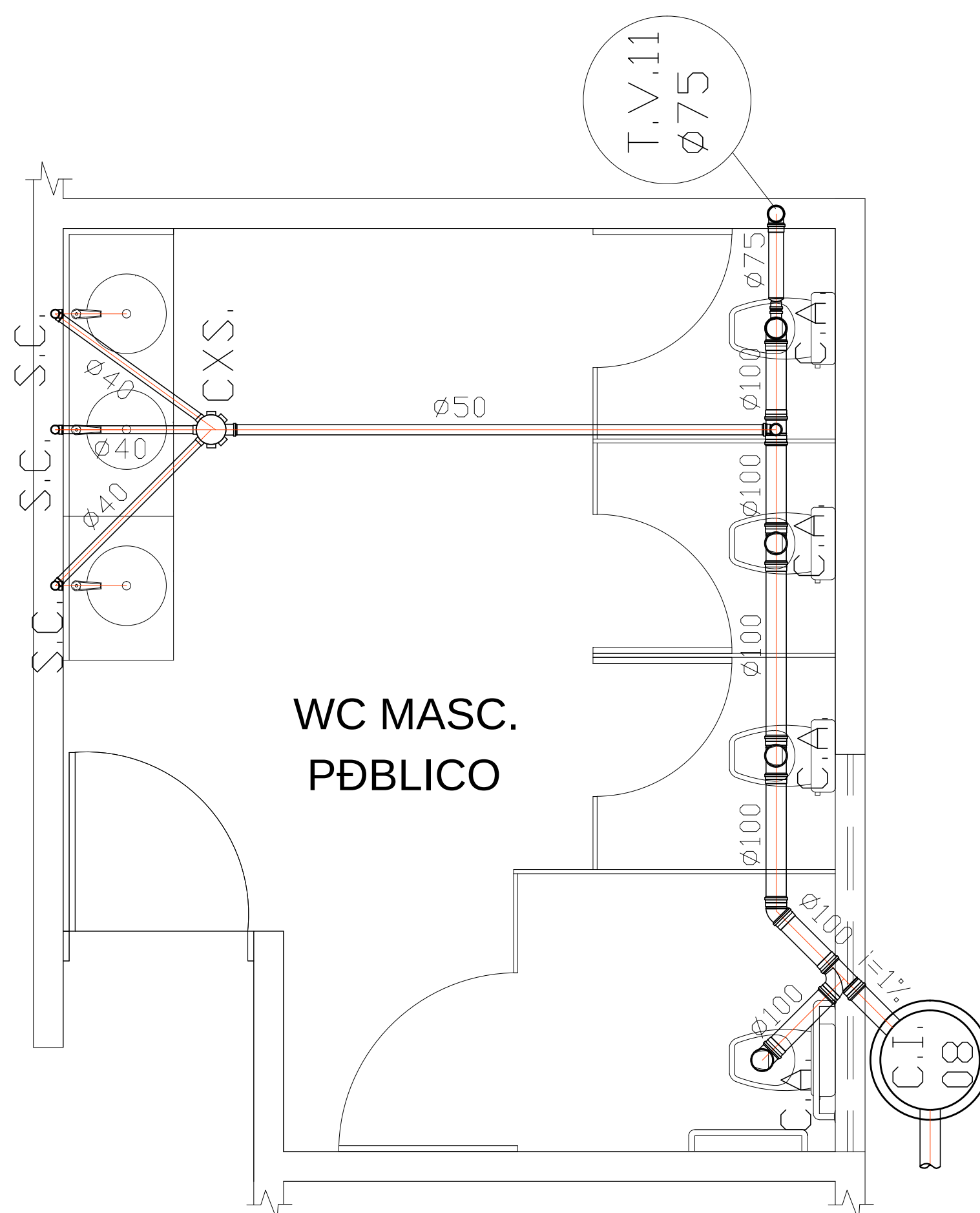
DETALHE 9 ESC. -----1/25
